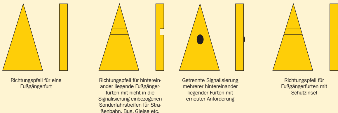
Taktile Zusatzinformationen an der Ober- oder Unterseite des Anforderungstasters (nach RiLSA)
