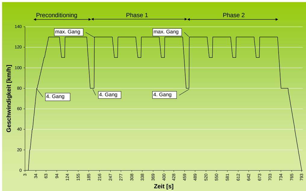
Abbildung 2: ADAC Autobahnzyklus
