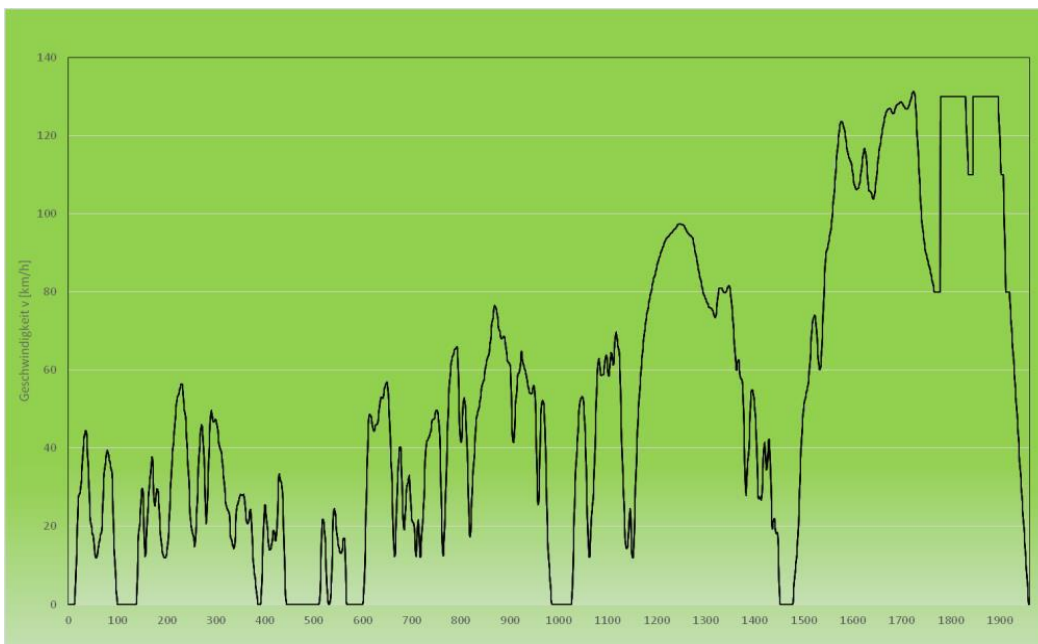
Abbildung 3: ADAC Elektrozyklus
