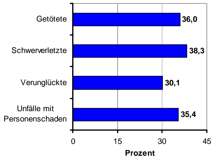
Anteil der Abkommensunfälle außerhalb von Ortschaften 2010
